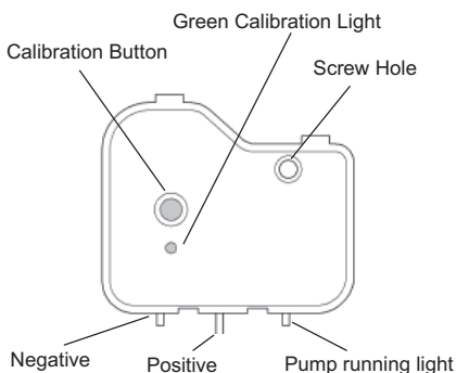
Fig 3: Watermaster® IC
